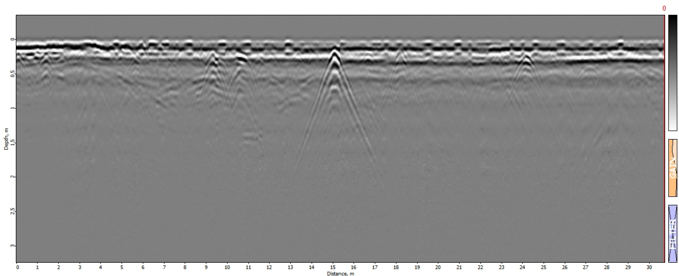
Georadaru darytas profilis, jame nustatyti po žeme esantys objektai (profilį sudarė S. Lozovskis)
